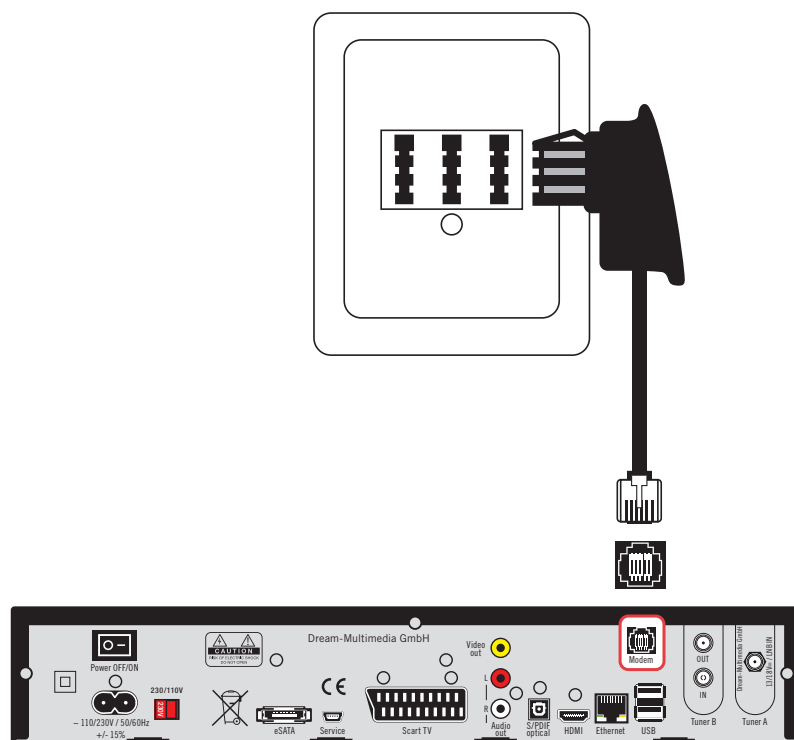
Modem anschließen
