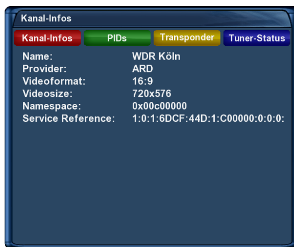
Kanal-Informationen
