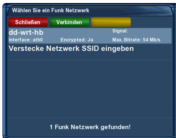
gefundene WLAN-Netzwerke
